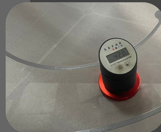
เครื่องวัดความตึงตะแกรง
