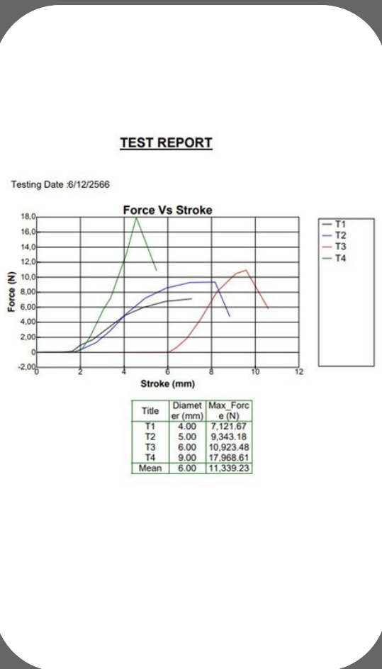
ใบ Cer. ทดสอบแรงดึง / แรงเฉือน
